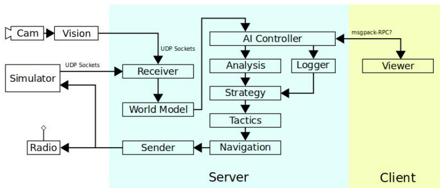
Fig. 7. AI System
