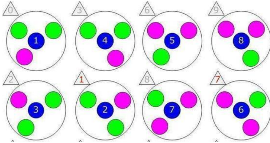
Fig. 16. Blobs Model
