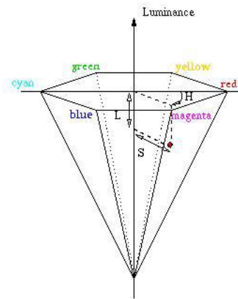
Fig. 12. Color Model
